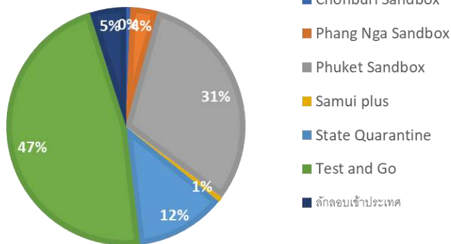
กราฟแสดงจำนวนของผู้ติดเชื้อแบ่งตามชนิดของการเข้ามา
