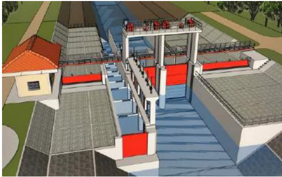
ภาพจำลองฝายพับได้ ภายหลังการก่อสร้างแล้วเสร็จ
